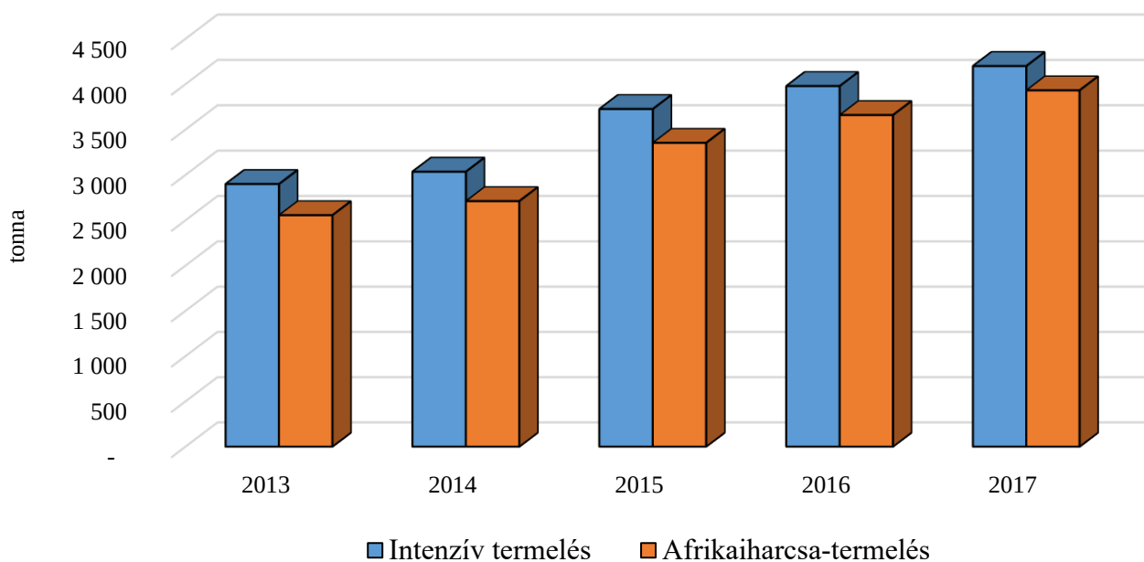
8. ábra: Afrikai harcsa mennyisége az intenzív termelésen belül 2013–2017 között
